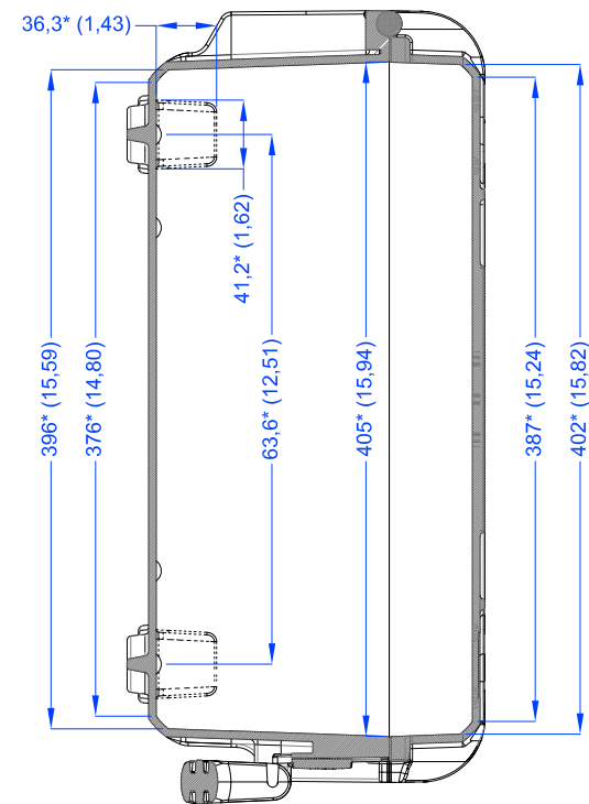
Sezione B-B Section B-B
